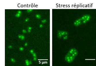
Figure 1 : Localisation de Hef::GFP
